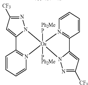
Os(fppz) 2 (PPh 2 Me) 2
