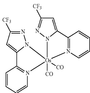
Os(fppz) 2 (CO) 2
